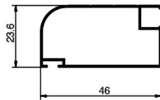
IF 553 Weight: 0.275 KG/M
