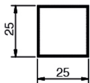
IF 106 Weight: 0.190 KG/M
