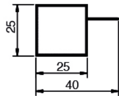
IF 111 Weight: 0.210 KG/M
