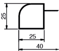
IF 123 Weight: 0.200 KG/M
