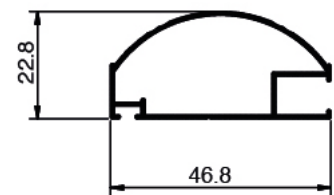
IF 560 Weight: 0.276 KG/M
