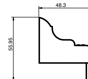
▶ IF 564 Weight: 0.340 KG/M
